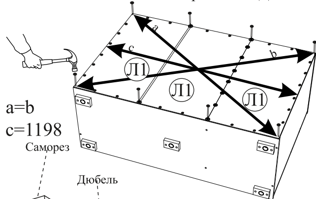
Рис.7 Прибивка ЛДВП
