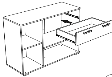
Рис.9 Установка выдвигающего ящика
